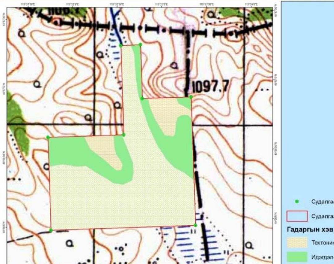
ДОРНОД АЙМГИЙН БАЯНДУН СУМЫН НУТАГТ БАЙРЛАХ “ЦЦ ЭРДЭС МАЙНИНГ” ХХК-ИЙН “ИХ НЭРГҮЙН АМ БА ТҮҮНИЙ БАРУУН САЛААНЫ АЛТНЫ ШОРООН ОРД АШИГЛАХ” ТӨСЛИЙН ТАЛБАЙН ГЕОМОРФОЛОГИЙН ЗУРАГ
