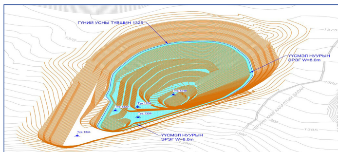
Зураг 1. Ил уурхайн газар хэлбэршүүлэлтийн изометр проекц
